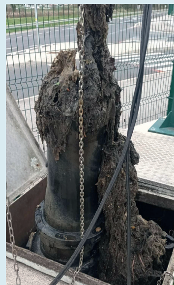
Zabite črpalke na kanalizacijskem črpališču, največ težav povzročajo vlažilni robčki.
